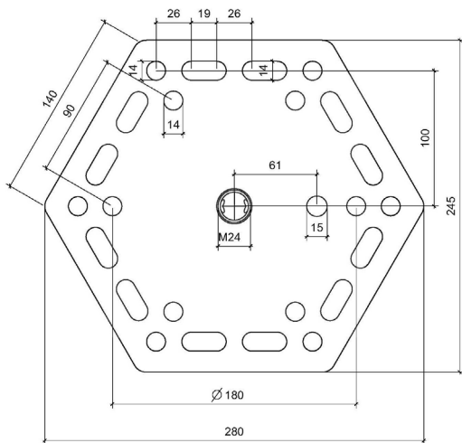
Flansch SW245/F15
