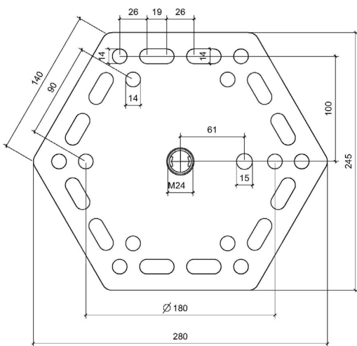
Bride SW245/F15
